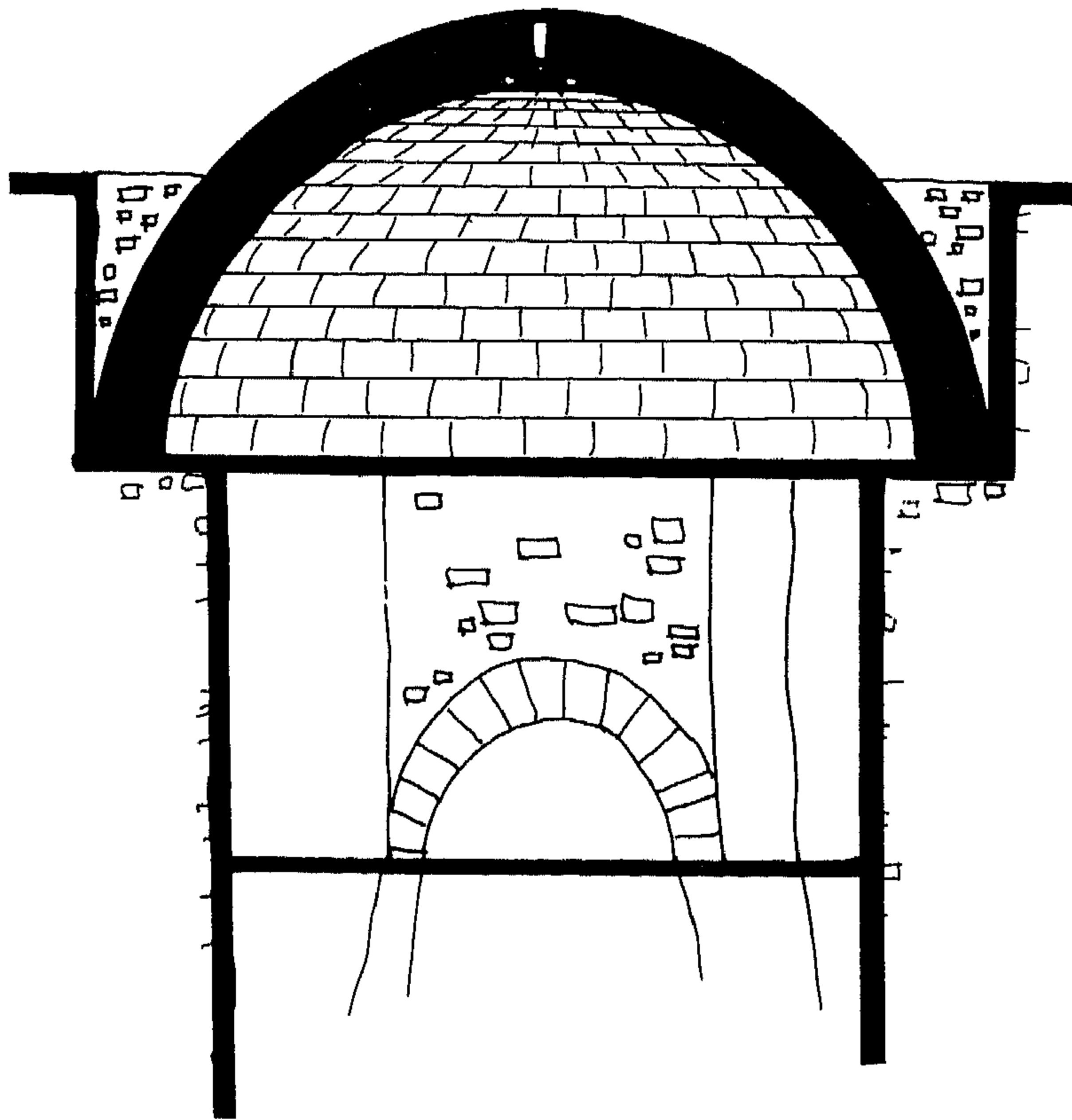
شكل (٢٩) مقطع لقبة العقد أسفل هيكل معبد أغسطس ببسبسية
